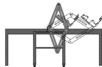
Figura 6. Prototipo de exoesqueleto: Movimiento para flexión y extensión. Página 60.
